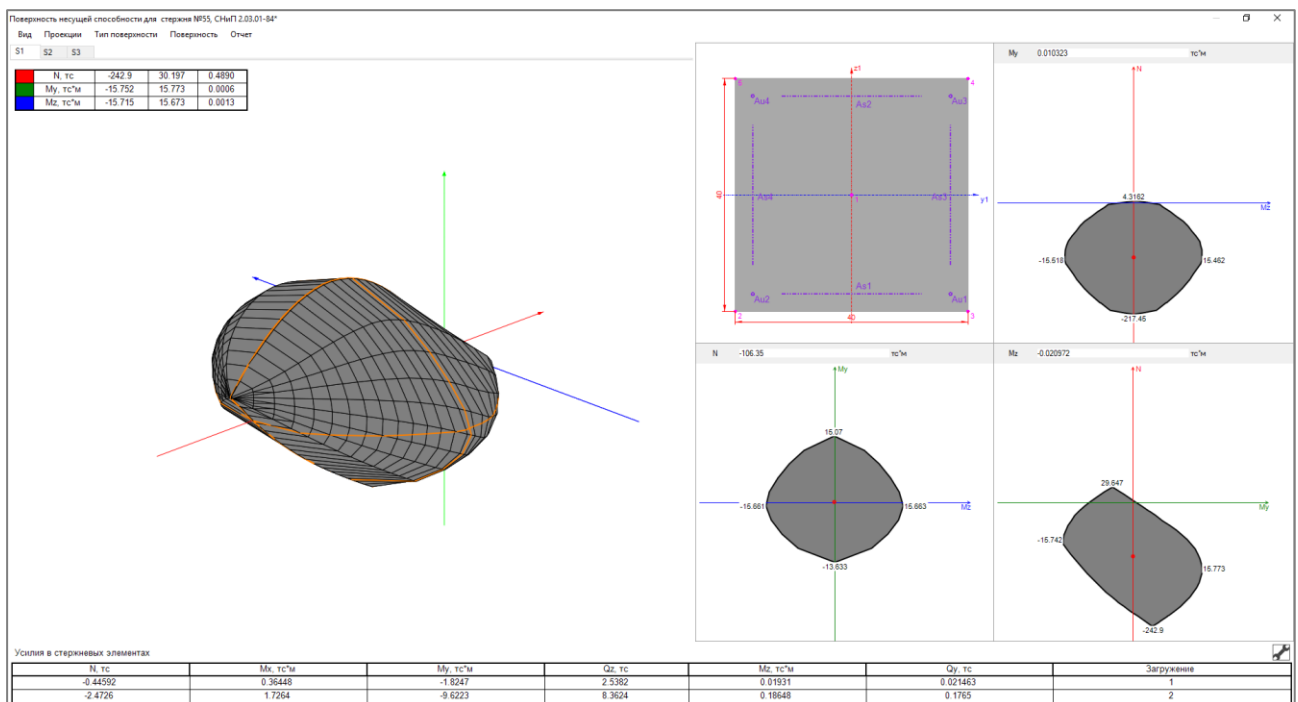
Рис. 8.47. Окно Поверхность несущей способности
