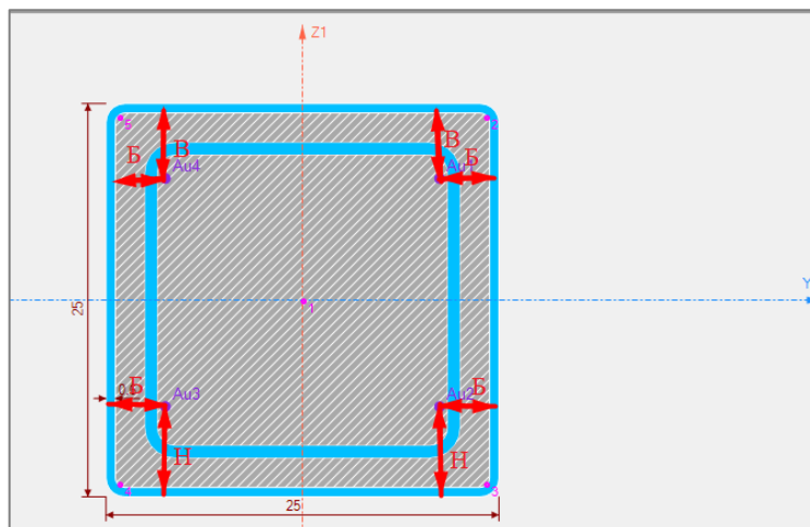
Рис. 8.12. Привязка центра тяжести арматуры к граням сечения швеллера: В — к верхней грани, Н — к нижней грани, Б — к боковой грани
